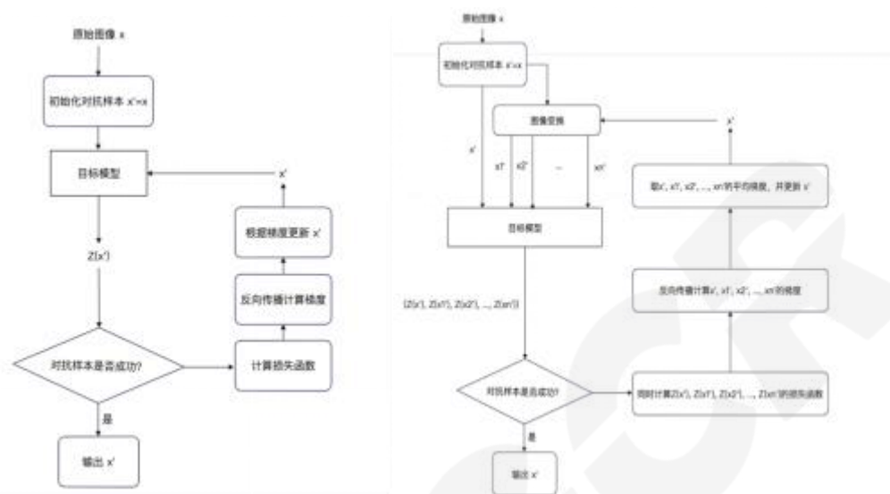
图 8 基于 PGD 的对抗样本生成算法（左）和 EOT 变体的对抗样本生成算法（右）
